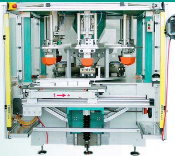
MM6 avec commande Siemens S7
